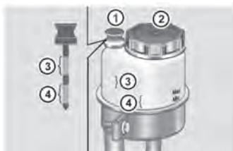
Reservatório de fluido da direção hidráulica
