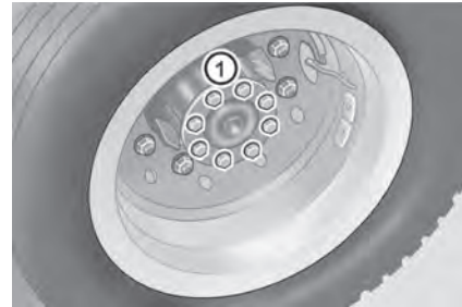
1- Parafusos de fixação da semi-árvore no cubo de roda (exemplo)
