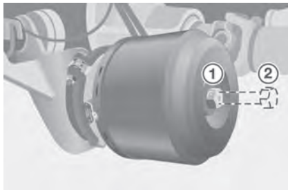
Parafuso de alívio do cilindro de mola acumuladora
