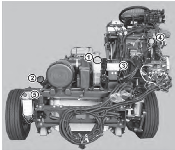
Pontos de manutenção (LO 916)
