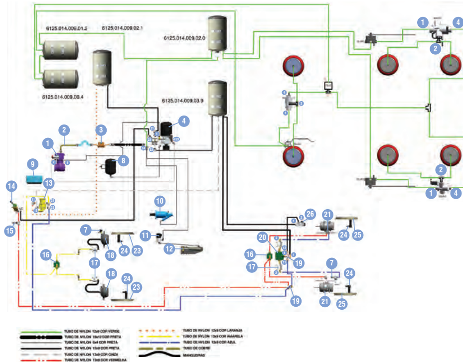
Esquema de Freio
